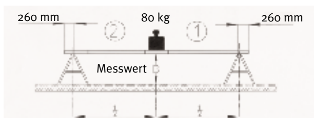
Bild 4: Belastete, umgesteckte Leiterteile mit Prüflast
